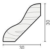
Profil 0516 30 x 30 x 2400 mm 20 Leisten je Bund
